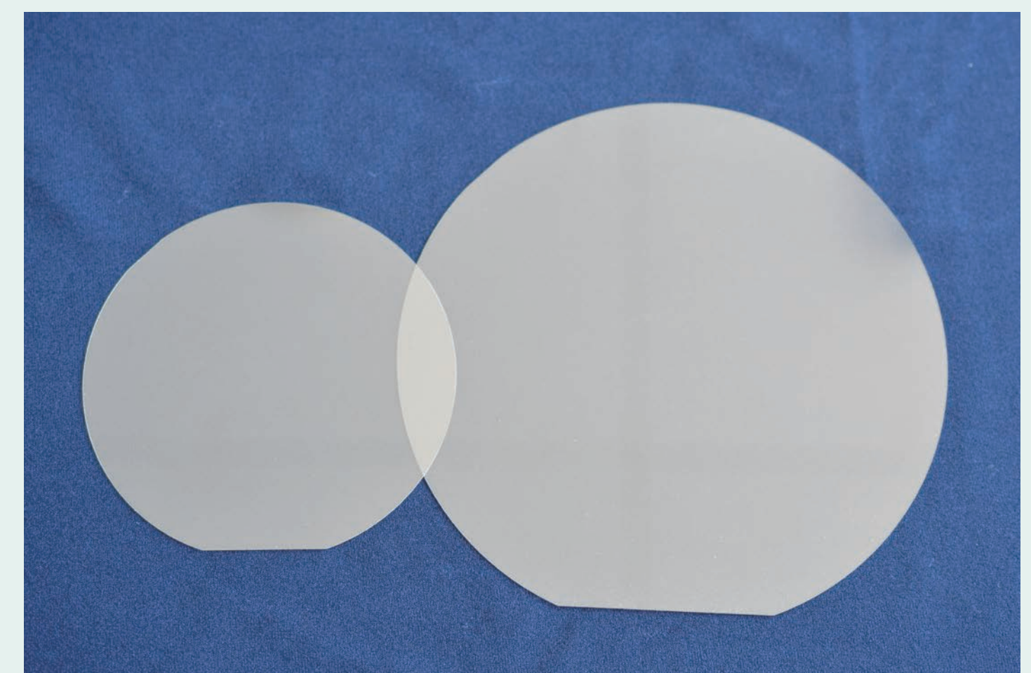
LiNbO 3 ウエハ (4inch、6inch)
